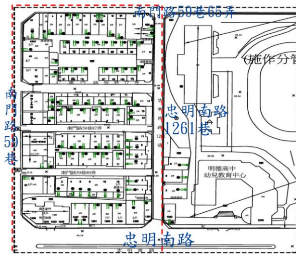
臺中市建成路系統污水下水道分支管網暨用戶接管工程（4）-台中路及忠明南路等鄰近區域 南區南門里附近地區
