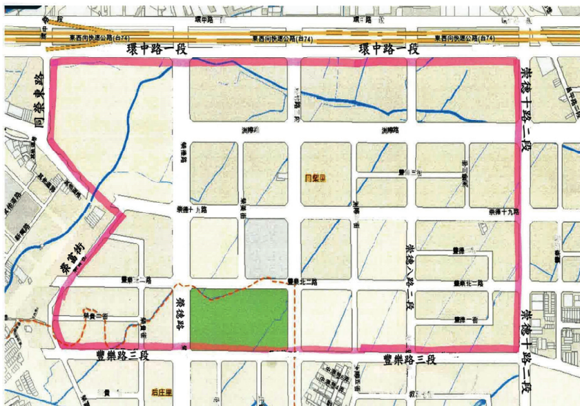
臺中市污水下水道公告可使用地區範圍圖 北屯區同榮里、后庄里等附近地區
