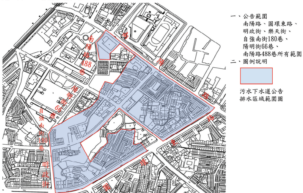
臺中市污水下水道公告使用區域之範圍圖
