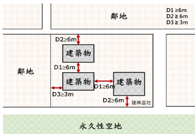
【附圖三之一】鄰棟間隔圖例
