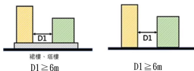
【附圖三之一】鄰棟間隔圖例
